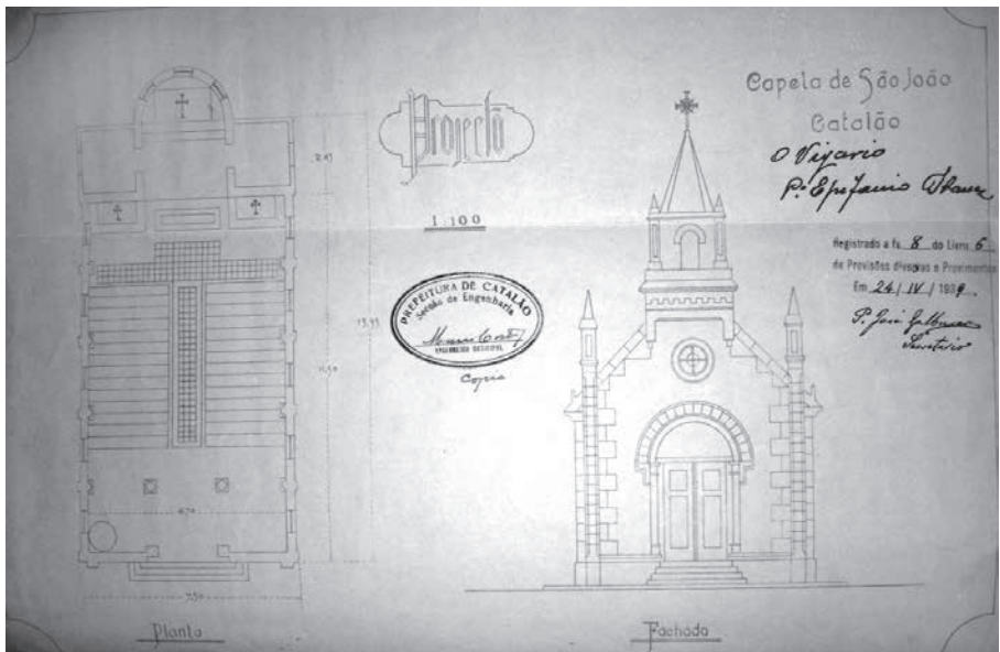
Planta da Igreja de São João Batista de Catalão
