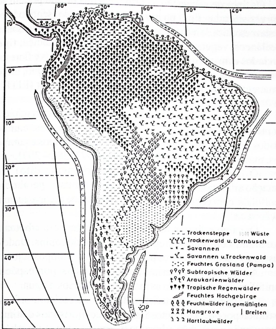
FIGURA 2 — Mapa da vegetação da América do Sul (SCHMIEDER, 1962 in WEBER, 1969). Tipos de vegetação: trockensteppe = estepe árida; wüste = deserto; trockenwald u. dornbusch = caatinga; savannen = savana; savannen u. trockenwald = cerrado; feuchtes grasland (pampa) = pampa; subtropische wälder = floresta subtropical; araukarienwälder = floresta de araucária; tropische regenwälder = floresta tropical úmida; feuchtes hochgebirge = floresta úmida andina; feuchtwälder in gemäßigten breiten = floresta temperada úmida subandina; mangrove = manguezal; hartlaubwälder = floresta seca.
